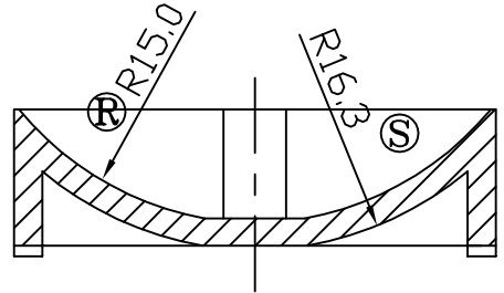
A-A截面图
