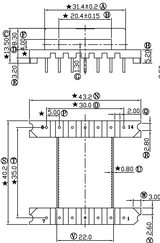
共B-1507模架
